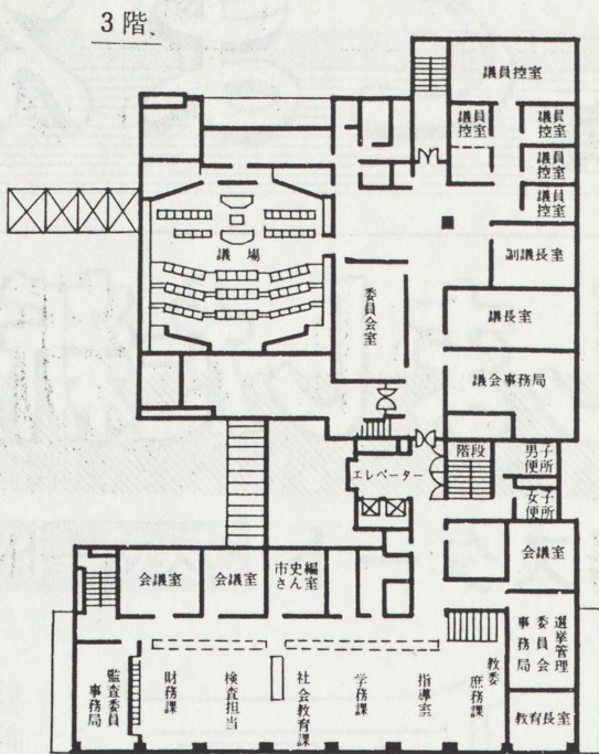
新庁舎平面図
